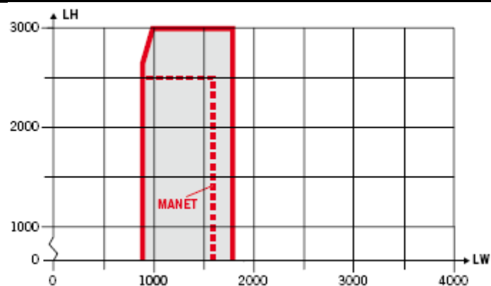
ST-ES 200 2D одностворчатая
