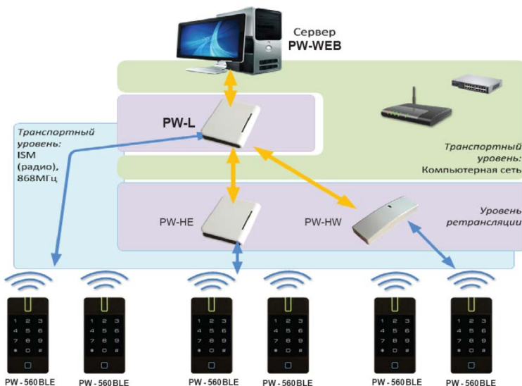
Рис 5. Построение системы беспроводных контроллеров
