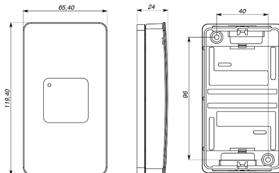
Рис 2. Габаритные размеры
