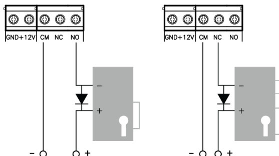
Рис.7. Подключение замков
