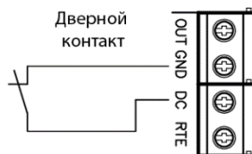
Рис.6. Подключение дверного контакта
