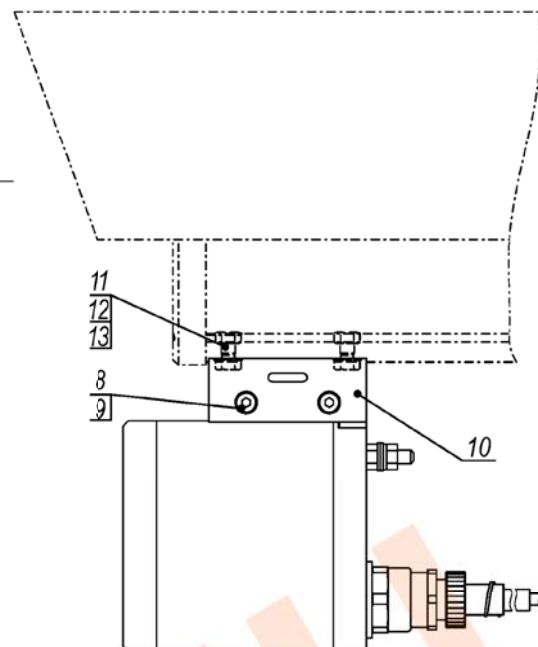
Рисунок 2 – Установка прожектора на видеокамеры в термокожухах ТГБ-4Г Ex, ТГБ-4Р Ex, ТГБ-4Г Ex IIC и ТГБ-4Р Ex IIC
