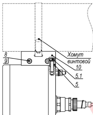
Рисунок 3 – Установка прожектора на видеокамеры других типов
