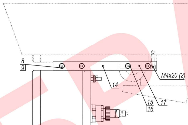
Рисунок 4 – Установка прожектора на видеокамеры в термокожухах ТГБ-4М Ex и ТГБ-4М Ex IIC
