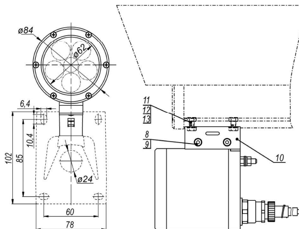
Рисунок 2 – Установка прожектора на видеокамеры в термокожухах ТГБ-4Г Ex, ТГБ-4Р Ex, ТГБ-4Г Ex IIC и ТГБ-4Р Ex IIC
