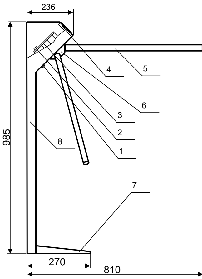
Рис. 1 Основные элементы турникета-трипода серии ТРТ-11-03
