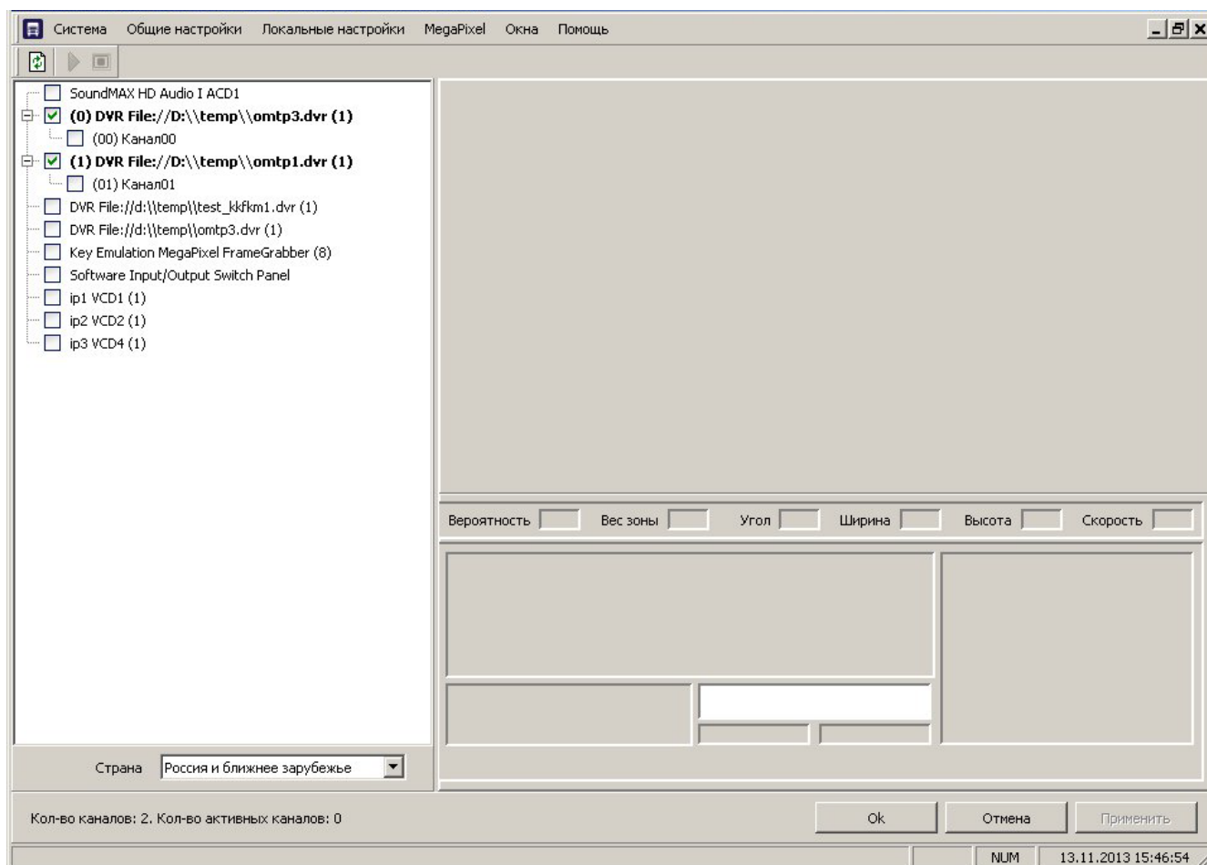
Рис. 4.4.1. Настройки распознавателя
