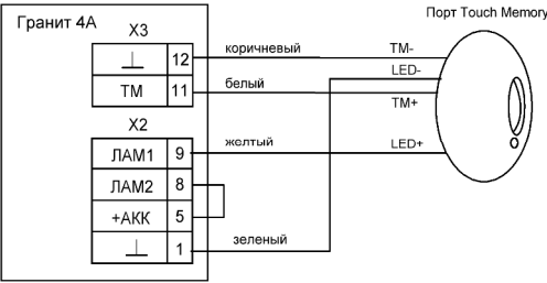
Рис. 1 Подключение порта Touch Memory
