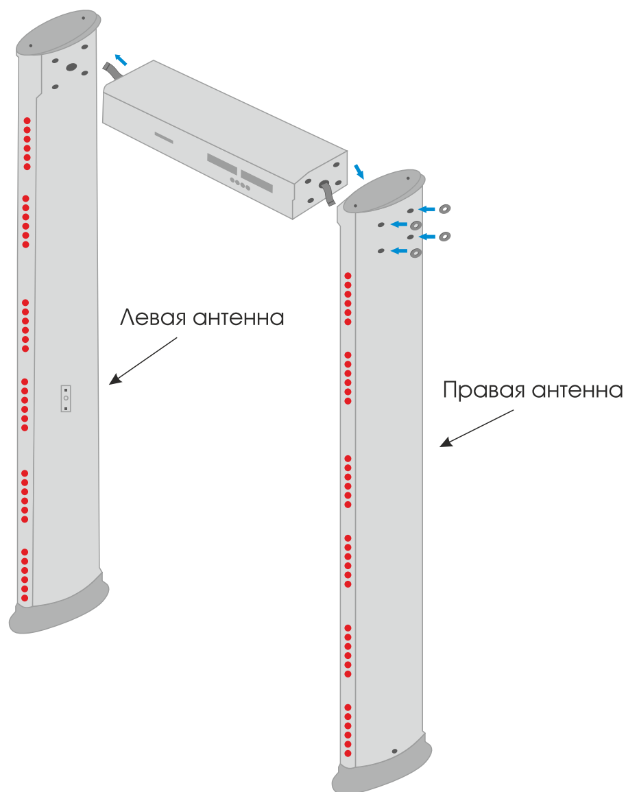
Рисунок 4. Сборка металлодетектора.
