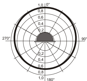
Рис.2 Схема подключения и диаграмма направленности звука оповещателя ПКИ-СП12.
