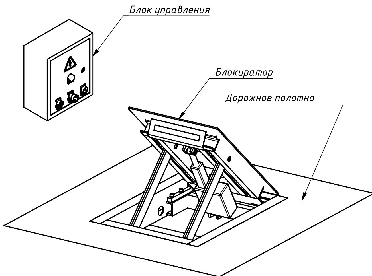
Рис.1 Общий вид
