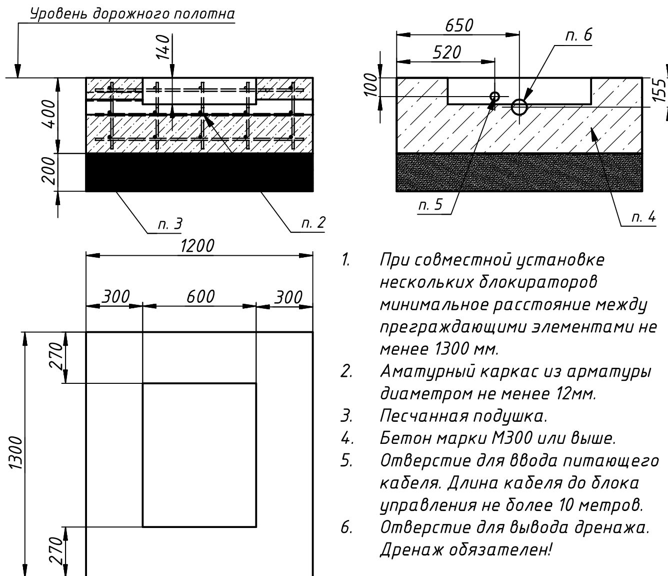
Рис.2 Габаритные размеры
