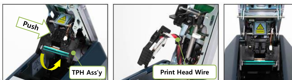
Рис. 104 Замена Печатной головки
