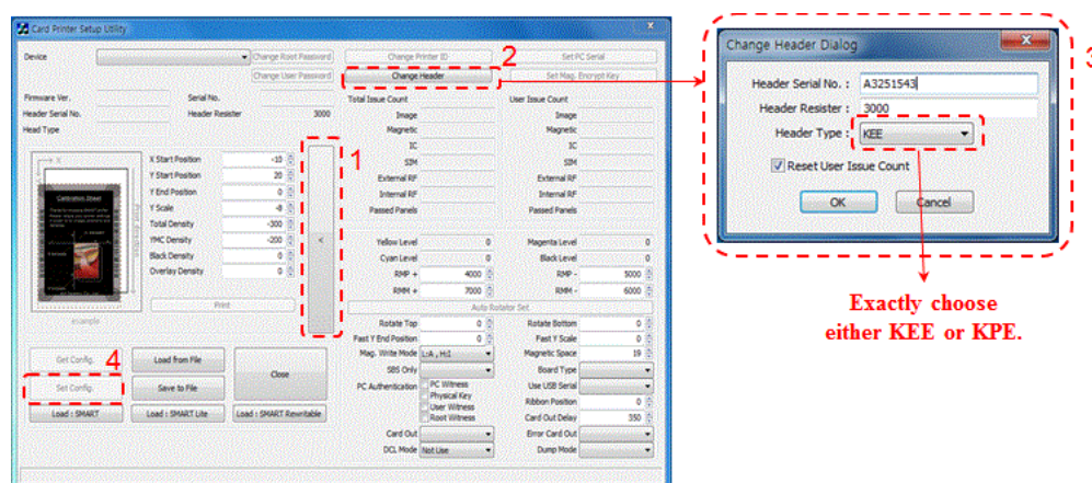
Рис. 113 Установка Печатной головки
