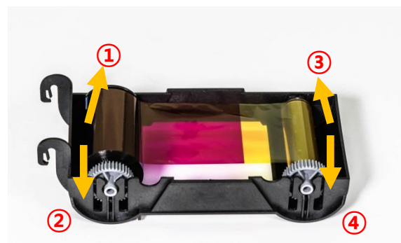
Figure 16 Загрузка ленты
