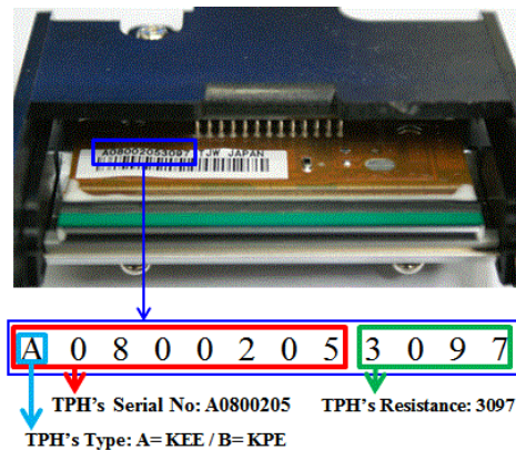
Рис. 10312 Термопечатная головка
