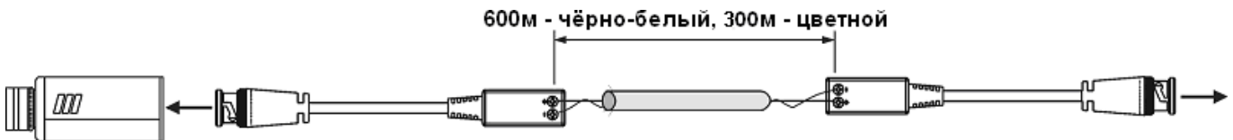
Рис.4 Подключение ТТР111VEL
