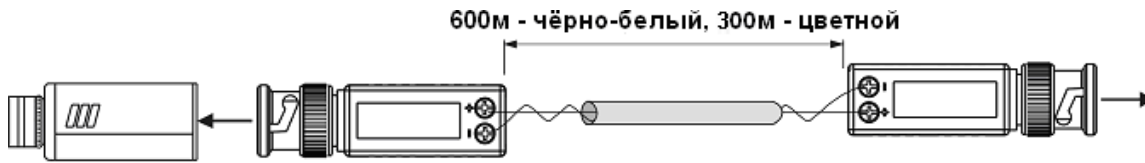
Рис.3 Подключение ТТР111VE
