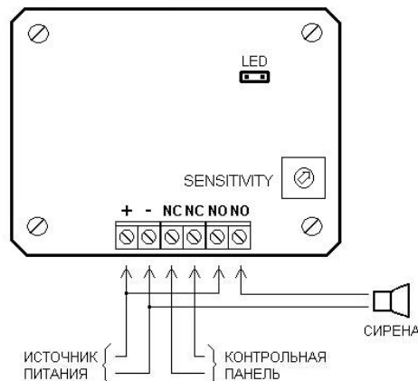
Рис. 1 Подключение извещателя
