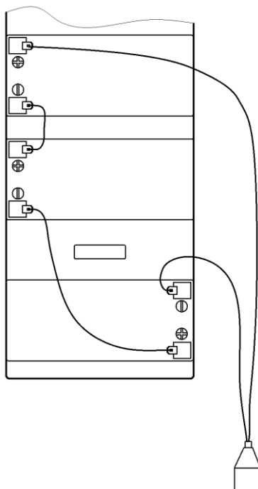
Рисунок 7 — схема соединений АКБ
