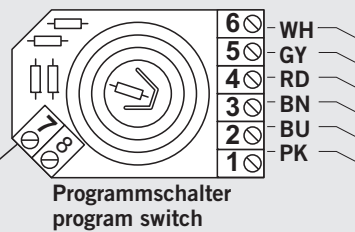
Programmschalter 5-stellig an ES 200 2D
