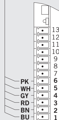
Steuerung ES 200 Grundmodul control system ES 200 basic module
