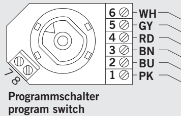
Programmschalter 5-stellig an ES 200
