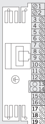
ES 200 FST / FIA Modul ES 200 FST / FIA module
