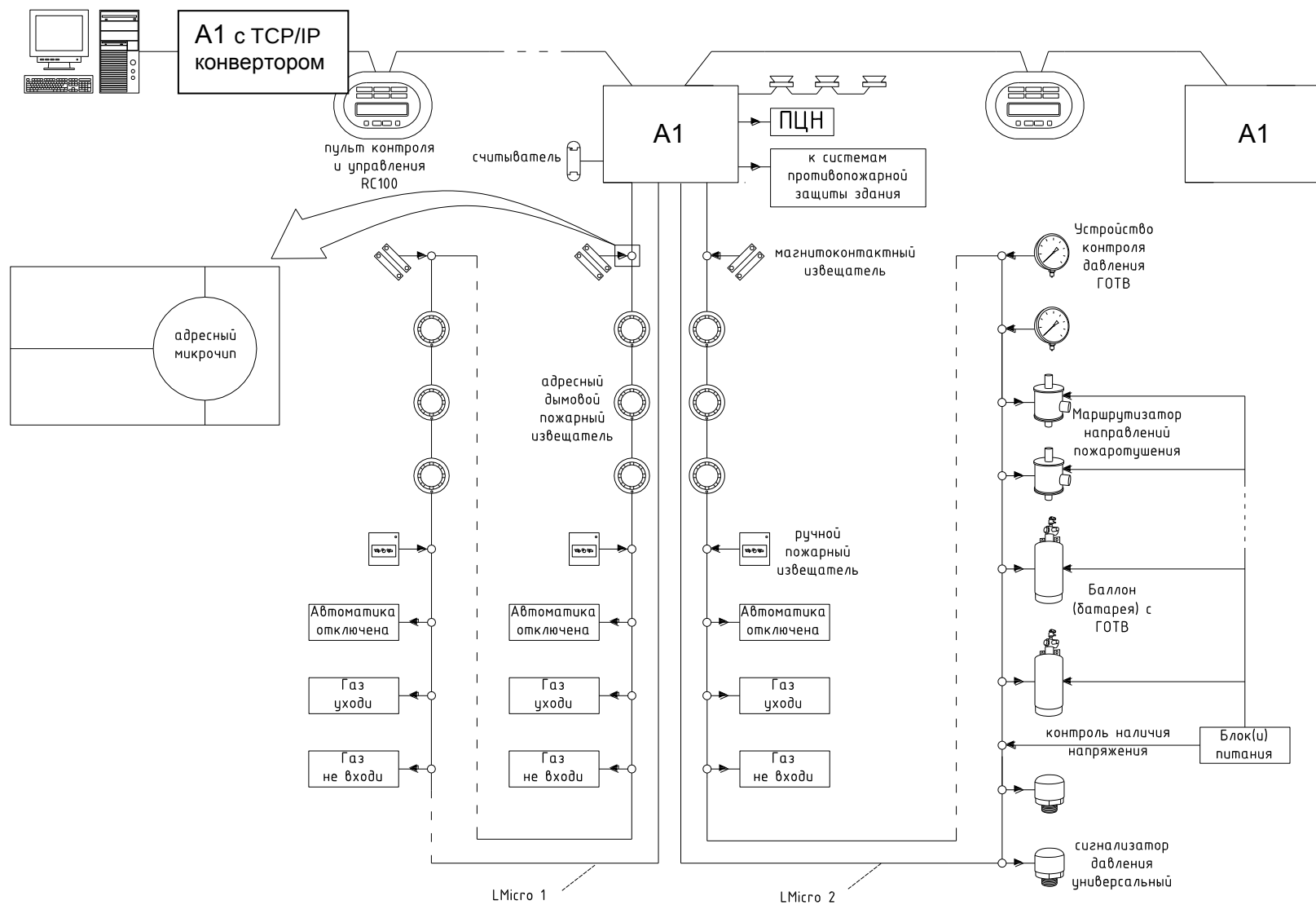
Рисунок 41. Адресная система ПС и УАПТ на базе контроллера А1
