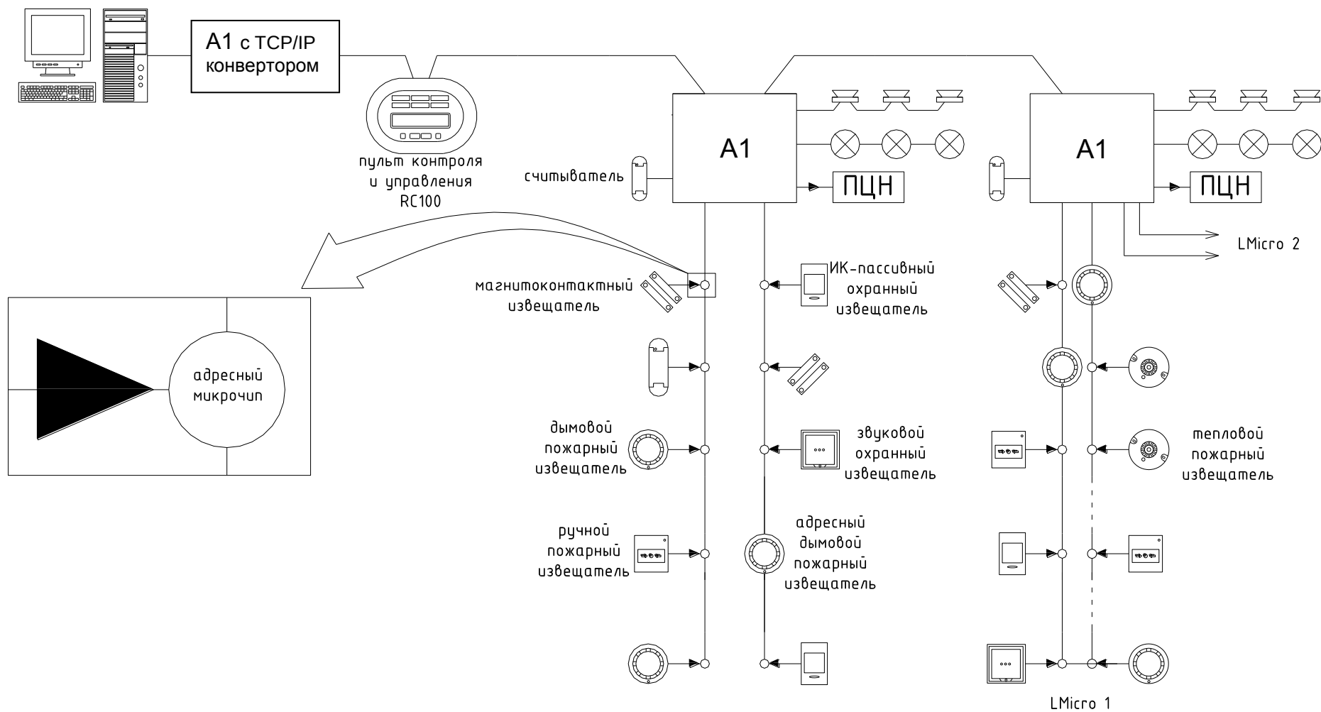
Рисунок 23. Пример адресной системы ОПС, построенной на базе контроллера А1
