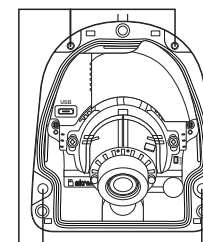
Крепежное отверстие
