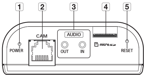
Передняя часть основного блока
