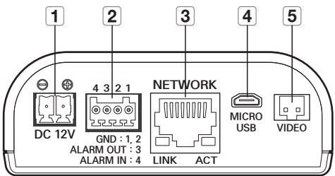
Задняя часть основного блока
