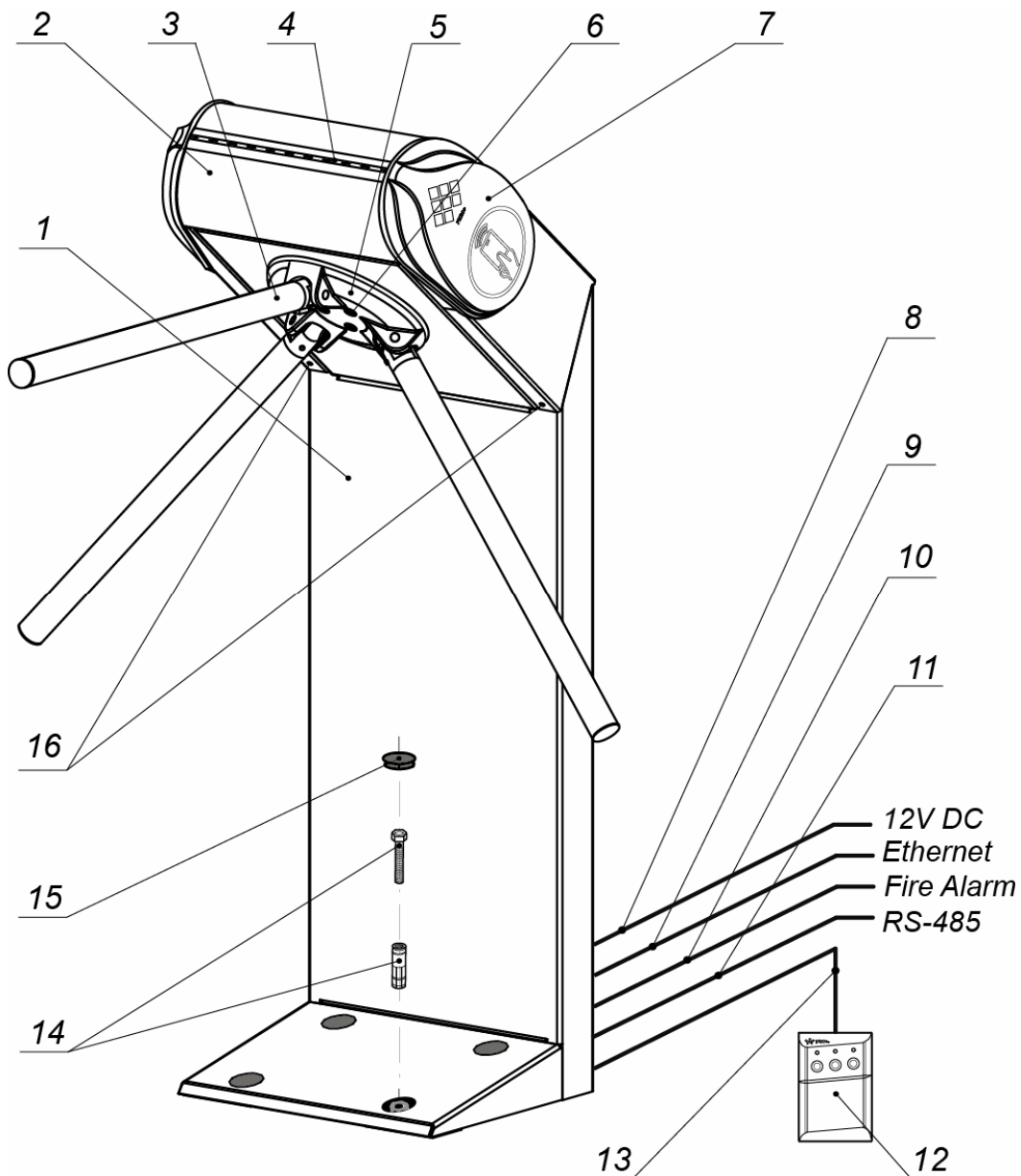
Рисунок 1. Устройство ЭП
