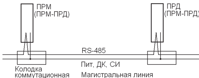
в) Вариант организации последовательного соединения
