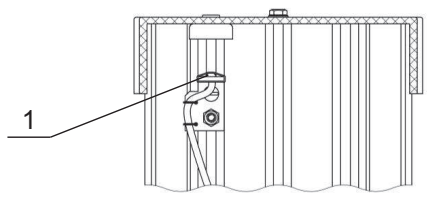
Рисунок 2.7 – Датчик вскрытия
