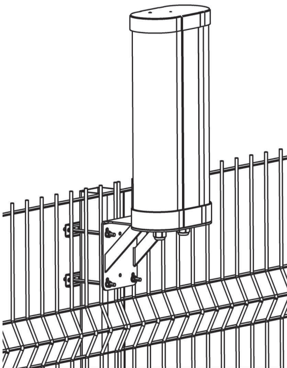
Рисунок 2.16 – Установка двухлучевой башни ПРМ-ПРД на стойках ограждения прямоугольного сечения
