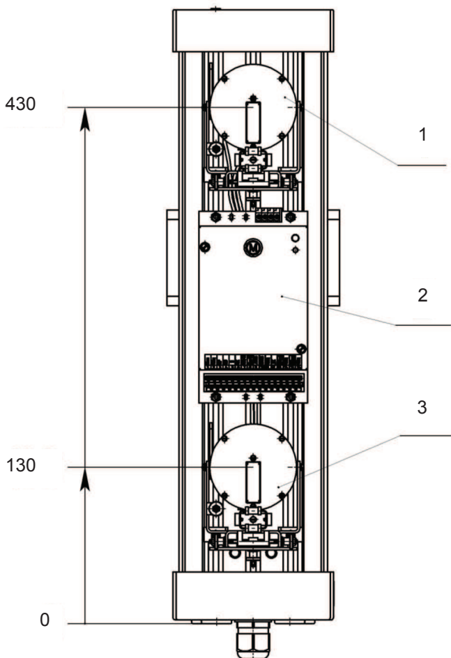
Рисунок 2.13 – Башня ПРД БАЖК.301317.009 (башня ПРМ БАЖК.301317.010, башня ПРД БАЖК.301317.021, башня ПРМ БАЖК.301317.022) со снятым защитным кожухом из поликарбоната
