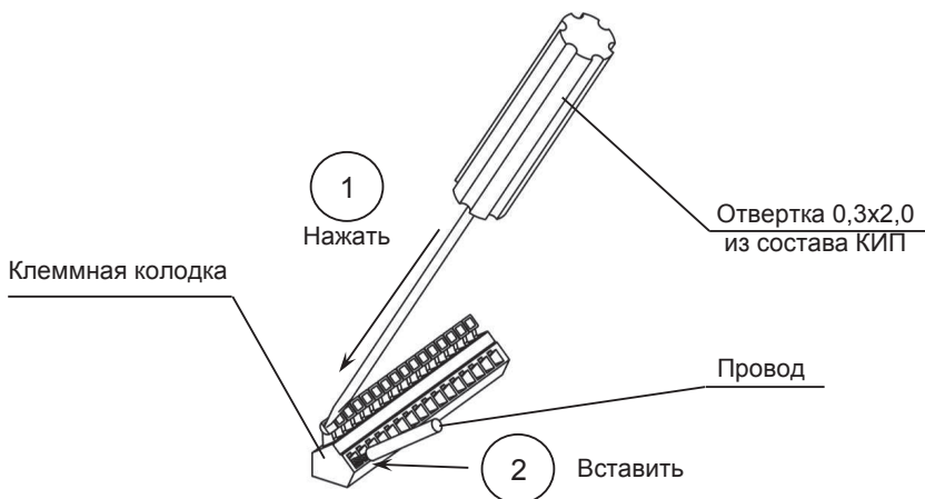
Рисунок 2.9 – Подключение проводов кабеля к клеммной колодке
