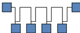
б) Последовательное соединение (рекомендуется)
