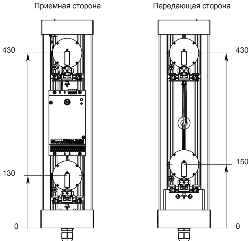
Рисунок 2.18 – Башня ПРМ-ПРД БАЖК.301317.012 (башня ПРМ-ПРД БАЖК.301317.024) со снятыми защитными кожухами из поликарбоната
