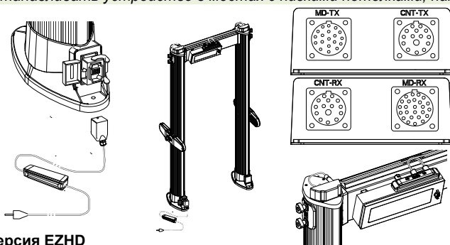
Версия EZHD
