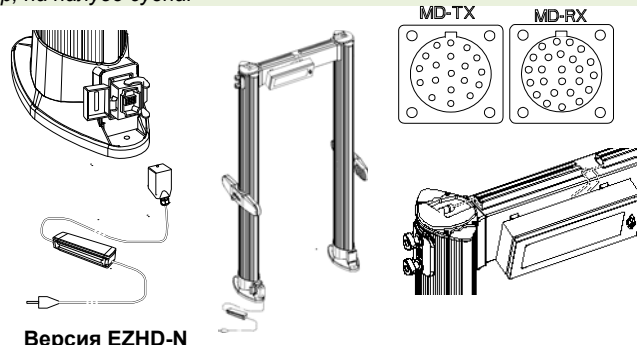
Версия EZHD-N
