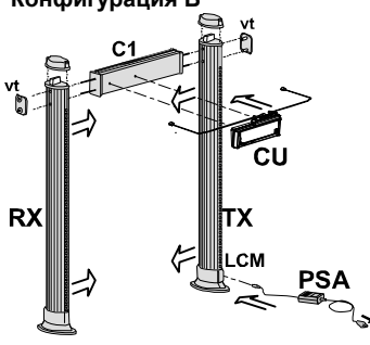
Конфигурация В
