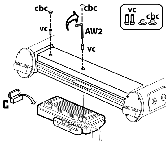
Конфигурация А
