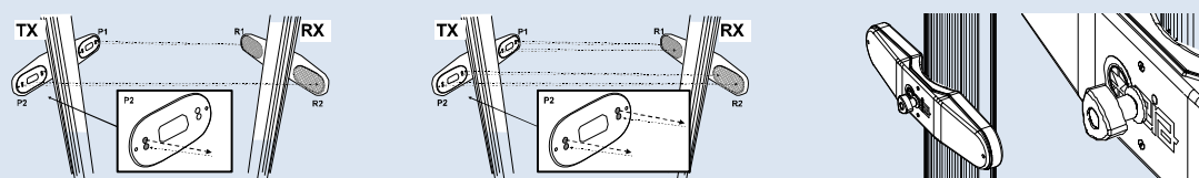
Колонная версия: 2-лучевые фотозлемента (код: 46982) 4-лучевые фотозлемента (код: 56109) [Для тяжелых условий]: версия для быстрой установки без инструментов
