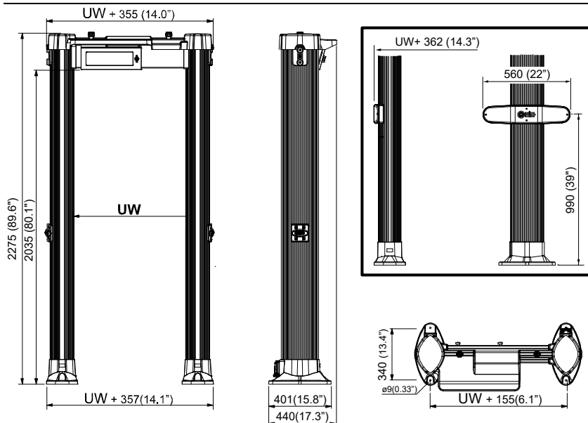
Эллиптические модели. Версия с защитными крышками. Размеры: UW = 720 мм (ВАРИАНТ: 820 мм).
