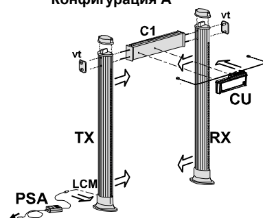
Конфигурация А
