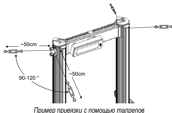
Пример привязки с помощью талрепов
