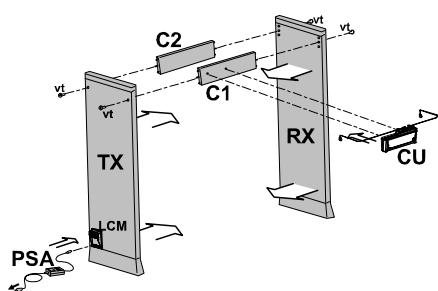
Конфигурация А
