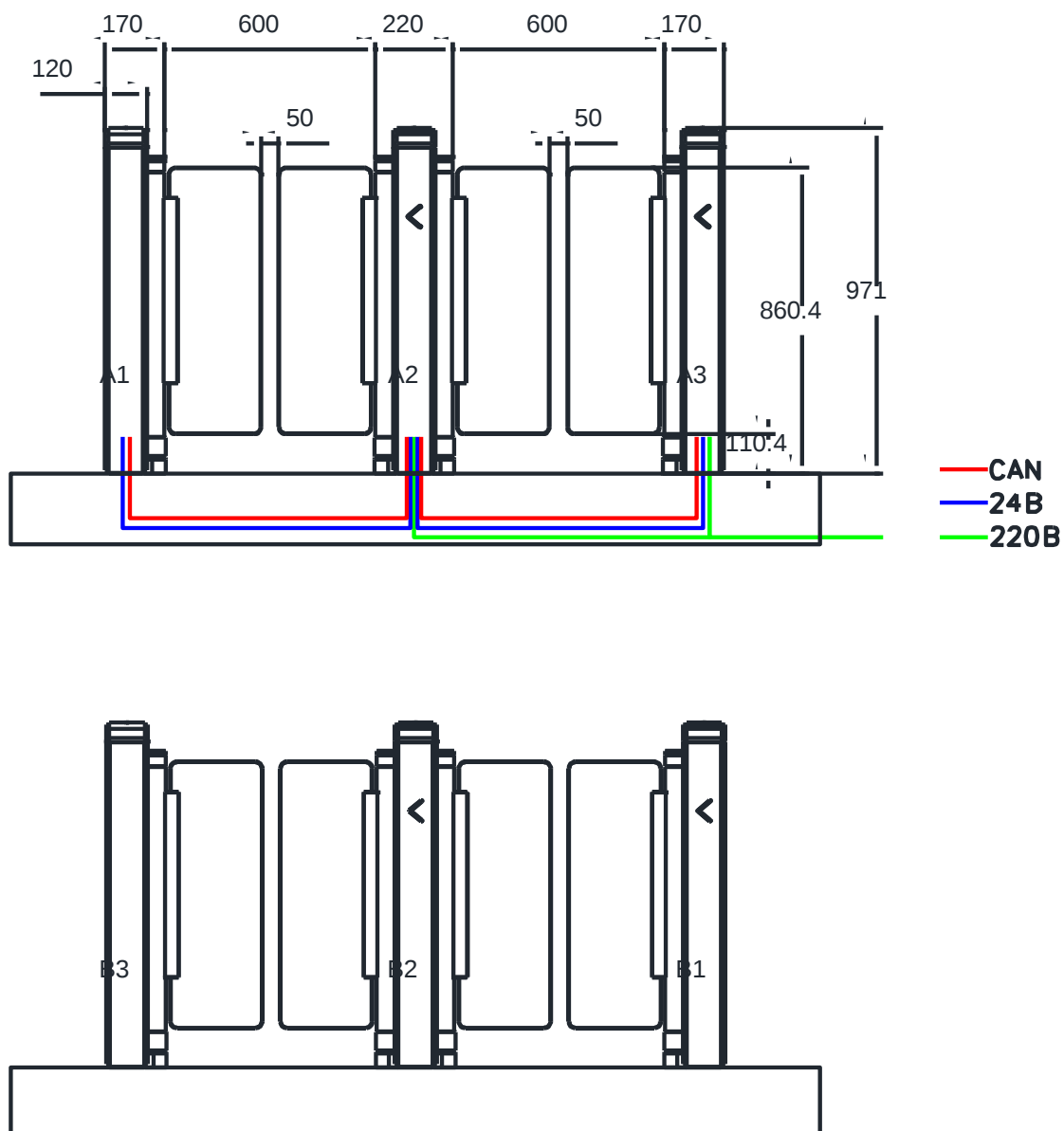
Рисунок 2 – Схема установки турникета
