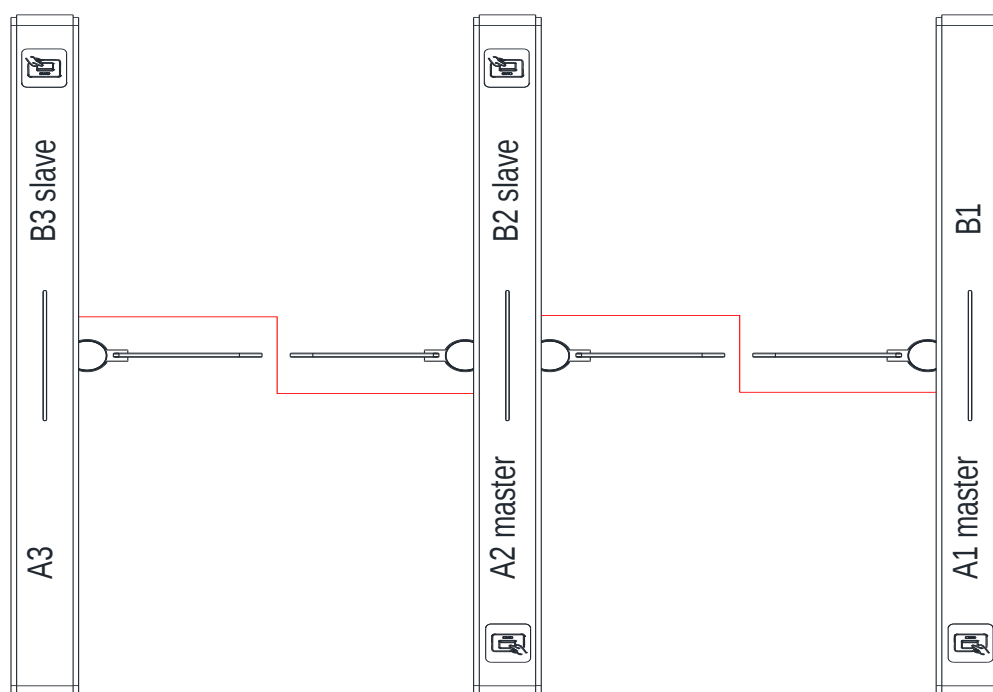
Рисунок 4 – Синхронизация плат управления Master и Slave
