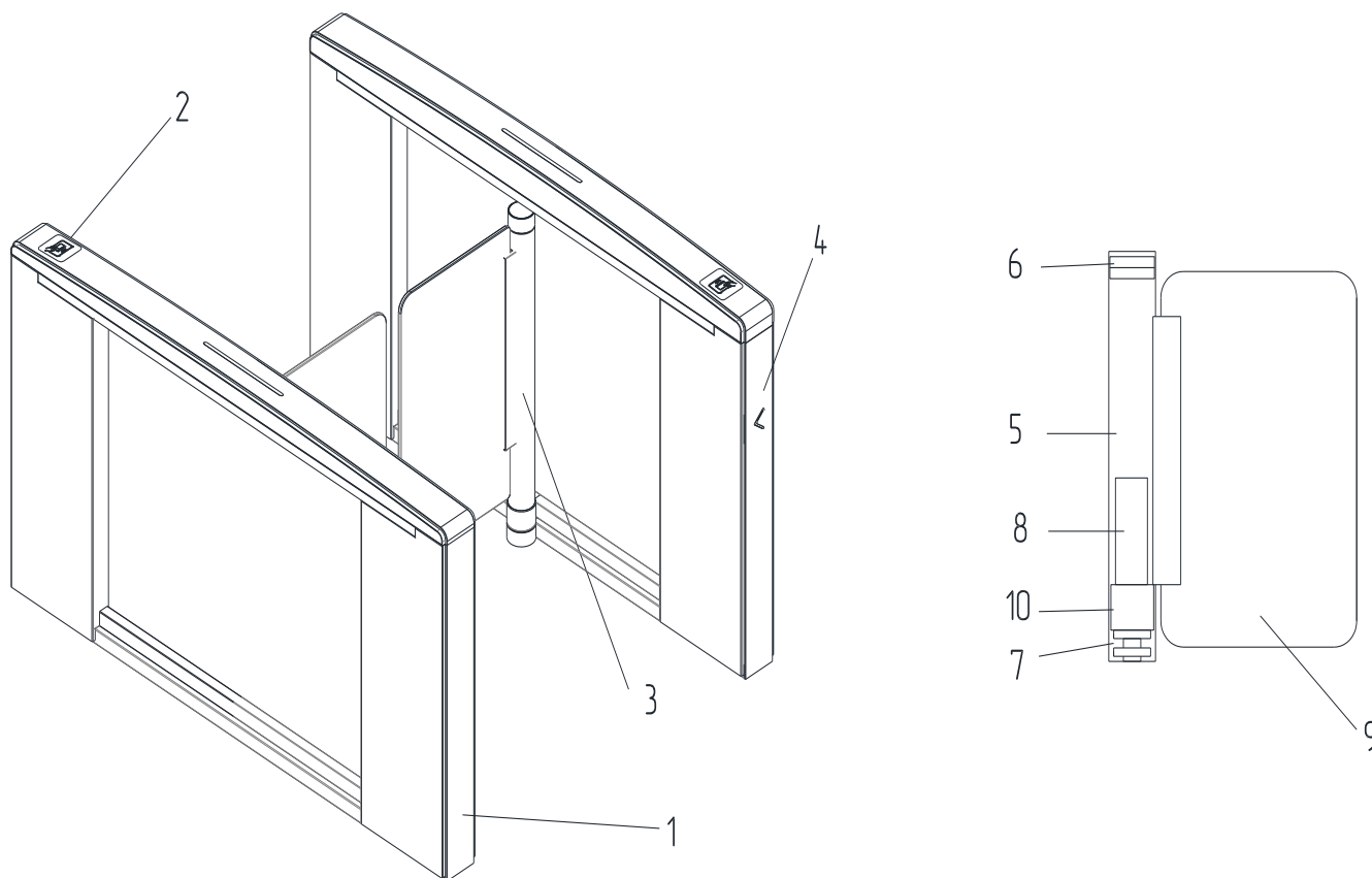
Рисунок 1 – Структура турникета:
