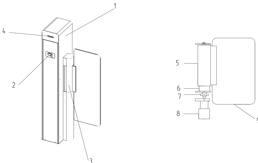
Рисунок 1 – Структура турникета:
