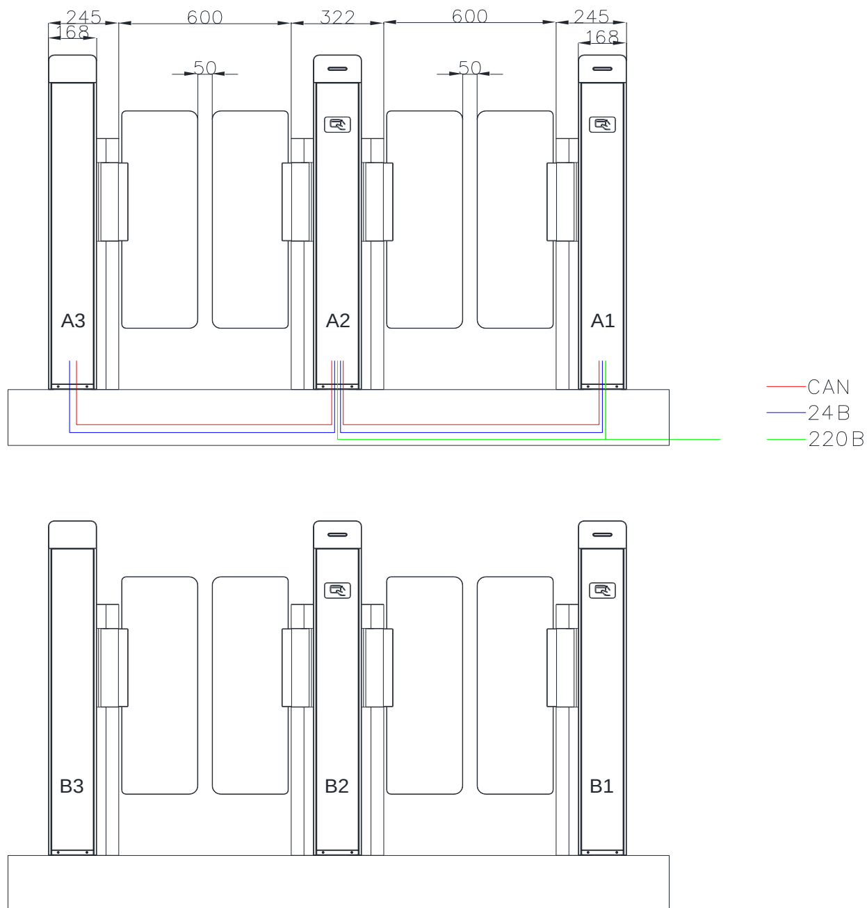
Рисунок 2 – Схема установки турникета
