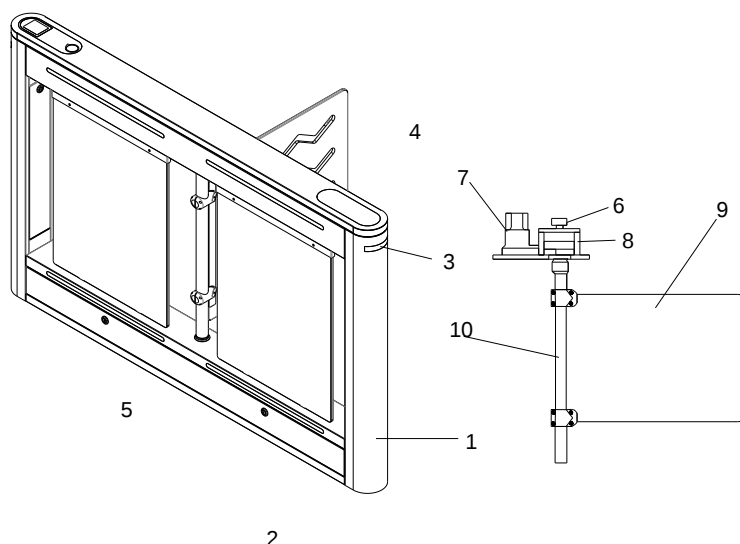
Рисунок 1 – Структура турникета:
