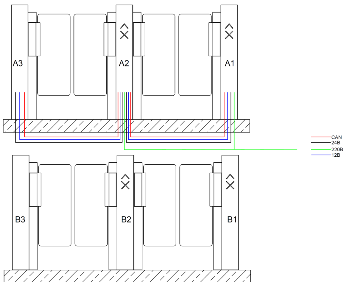
Рисунок 2 – Схема установки турникета
