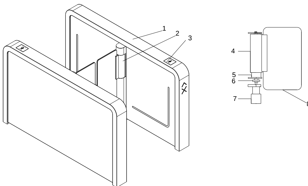
Рисунок 1 – Структура турникета:
