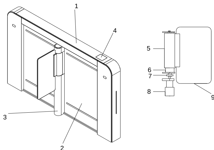
Рисунок 1 – Структура турникета:
