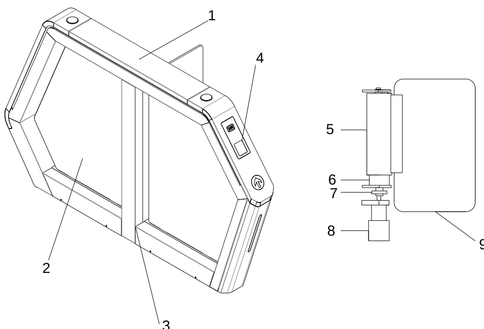
Рисунок 1 – Структура турникета:
