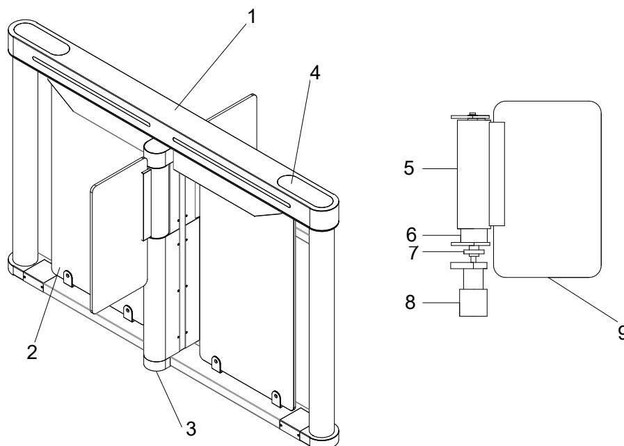
Рисунок 1 – Структура турникета:
