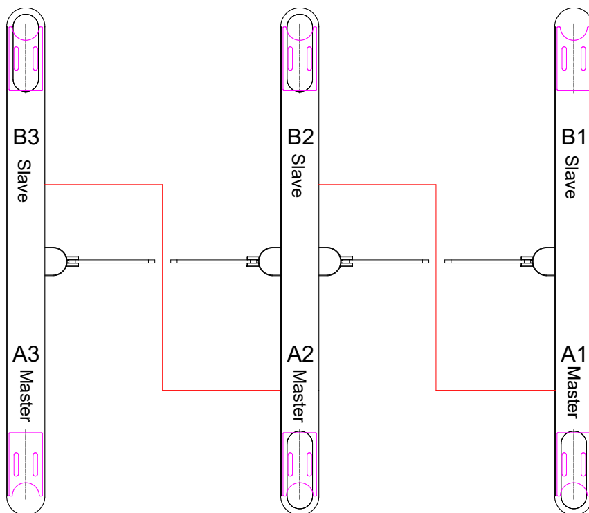
Рисунок 4 – Синхронизация плат управления Master и Slave
