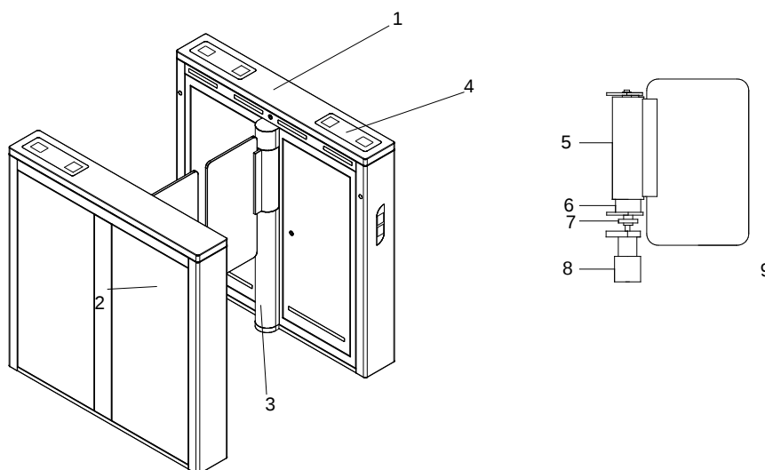
Рисунок 1 – Структура турникета:
