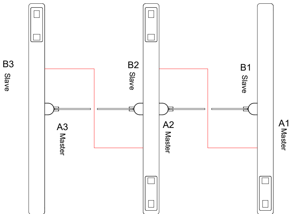
Рисунок 4 – Синхронизация плат управления Master и Slave
