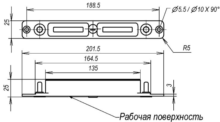
Рисунок 5 - Корпусная часть
