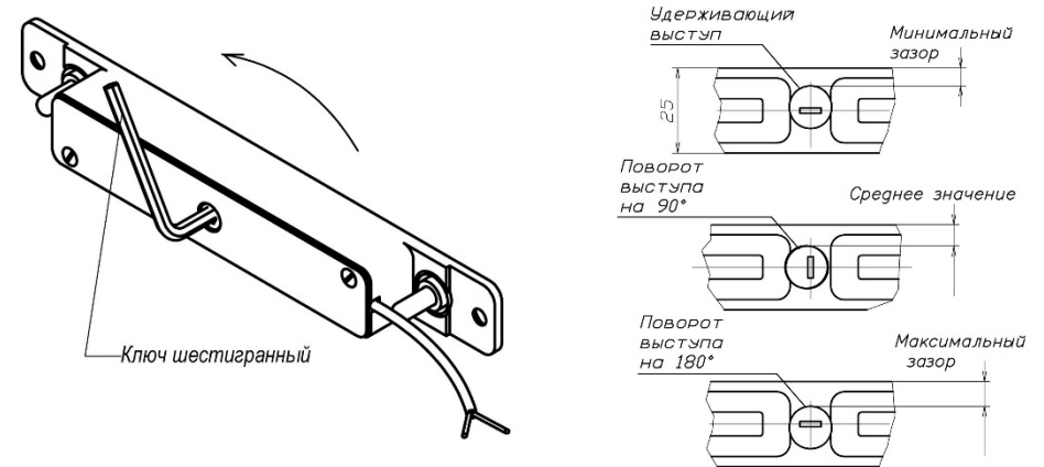
Рисунок 8 - Эксцентриковая регулировка зазора
