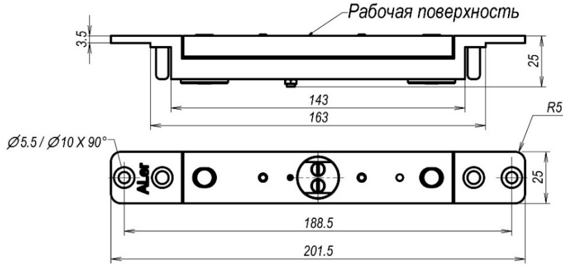
Рисунок 4 - Якорная часть
