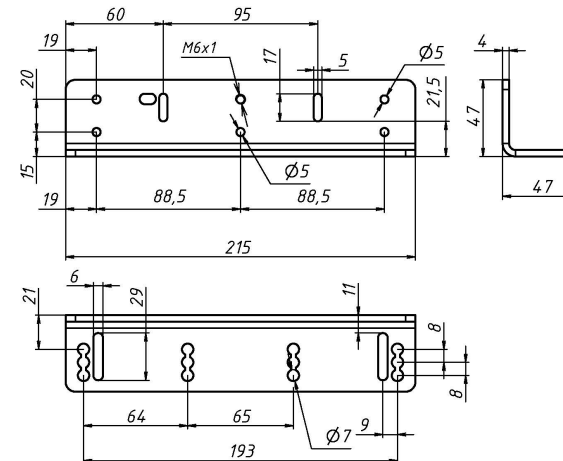
Рисунок 4 - Установка замка с монтажным комплектом МК AL-350FB-M-01
