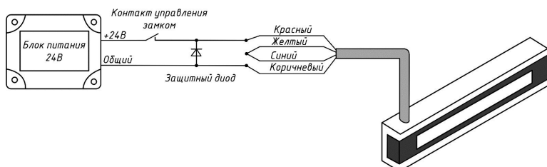
Рисунок 14 – Схема подключения замка при напряжении питания 24 В
