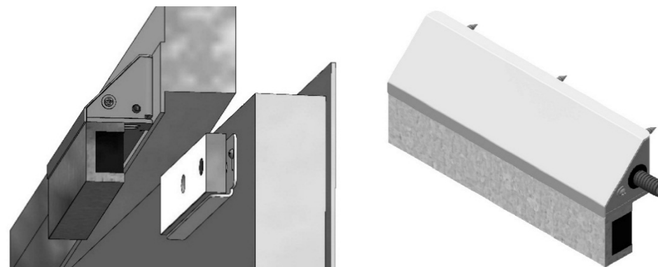
Рисунок 5 – Корпус с монтажным комплектом МК AL-350FB-M-02
