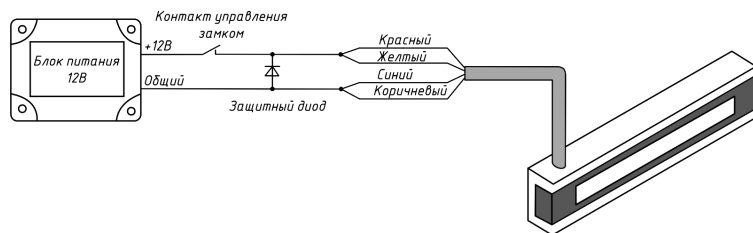
Рисунок 13 - Схема подключения замка при напряжении питания 12В
