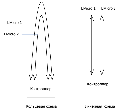
Рисунок 40. Варианты подключения адресных линий LMicro к контроллеру A1
