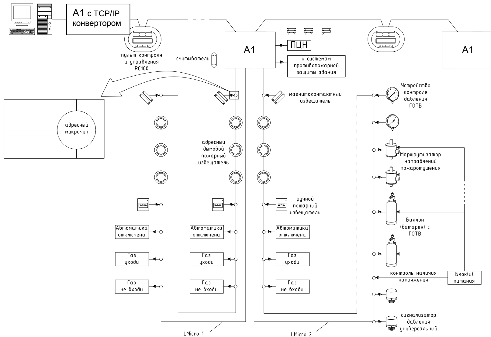
Рисунок 41. Адресная система ПС и УАПТ на базе контроллера А1
