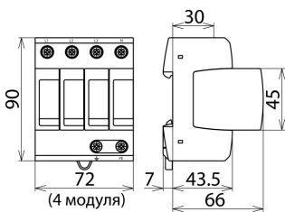
Размерный эскиз DG M TNS 275
