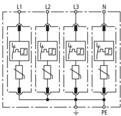
Принципиальная схема DG M TNS 275
