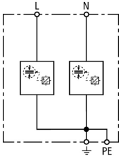
Принципиальная схема DSH TN 255
