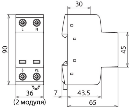
Размерный эскиз DSH TN 255
