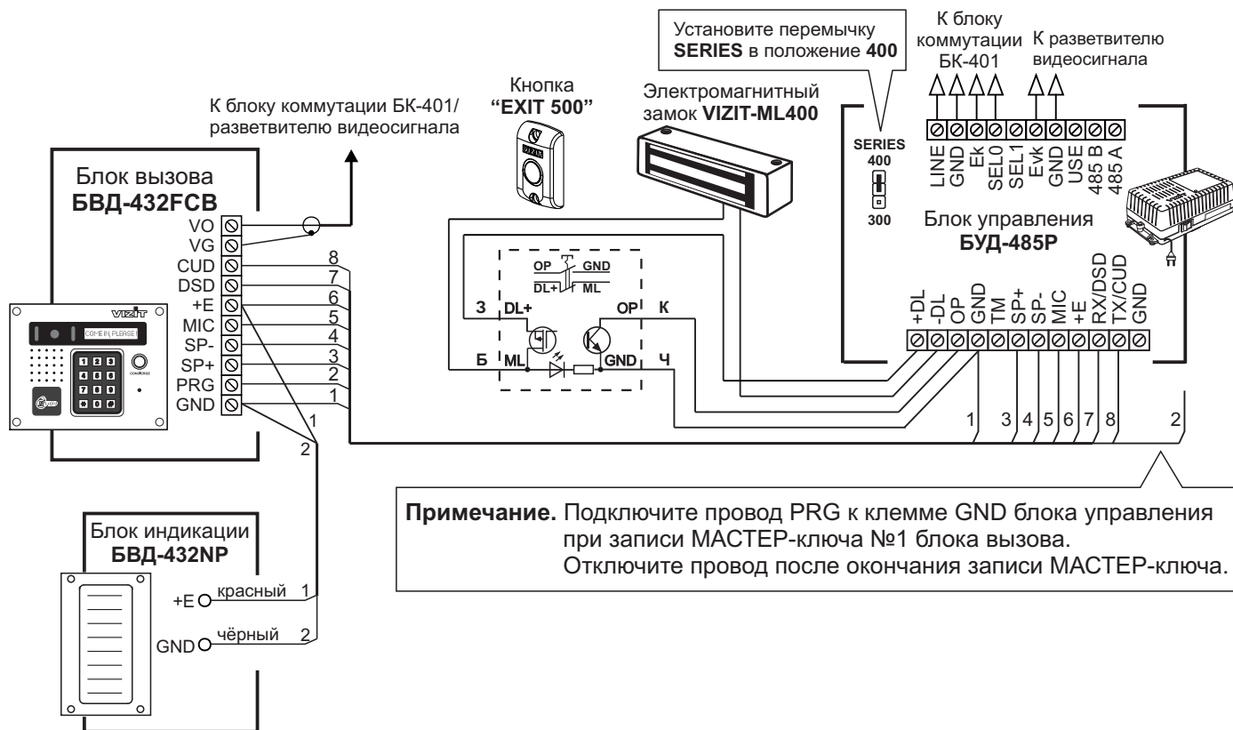
Рисунок 3 - Схема соединений блока вызова БВД-432FCB с блоком управления БУД-485P , блоком индикации БВД-432NP , электромагнитным замком VIZIT-ML400 и кнопкой “EXIT 500”
